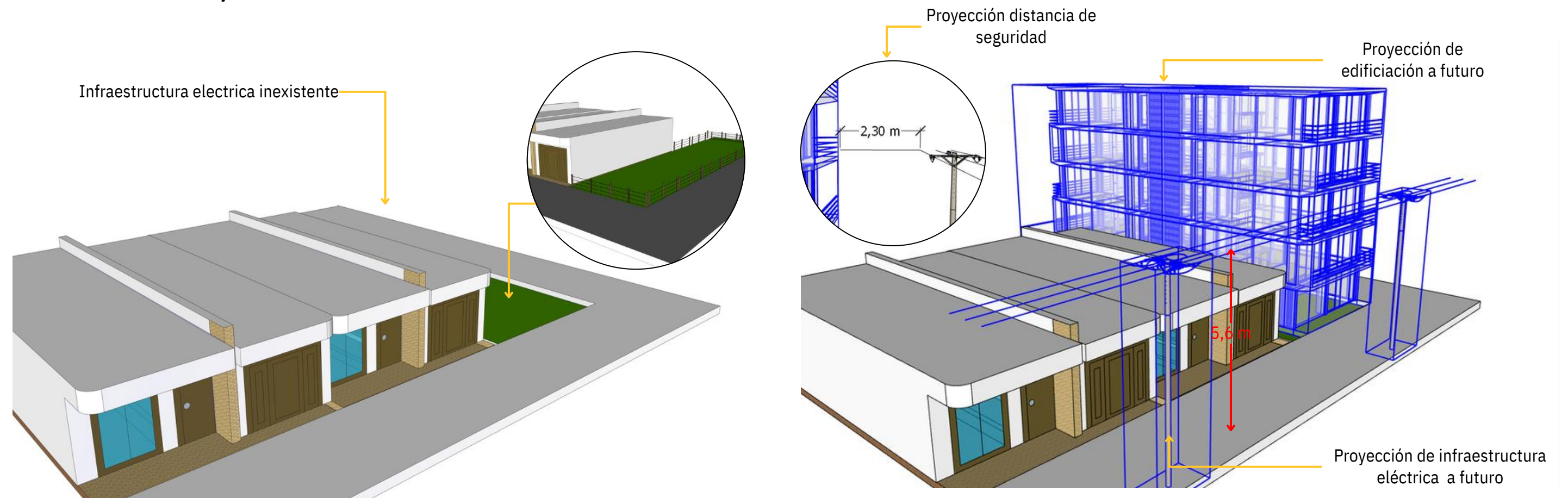
Figura 4. Distancias mínimas de seguridad en zonas con construcciones con infraestructura electrica inexistente.
