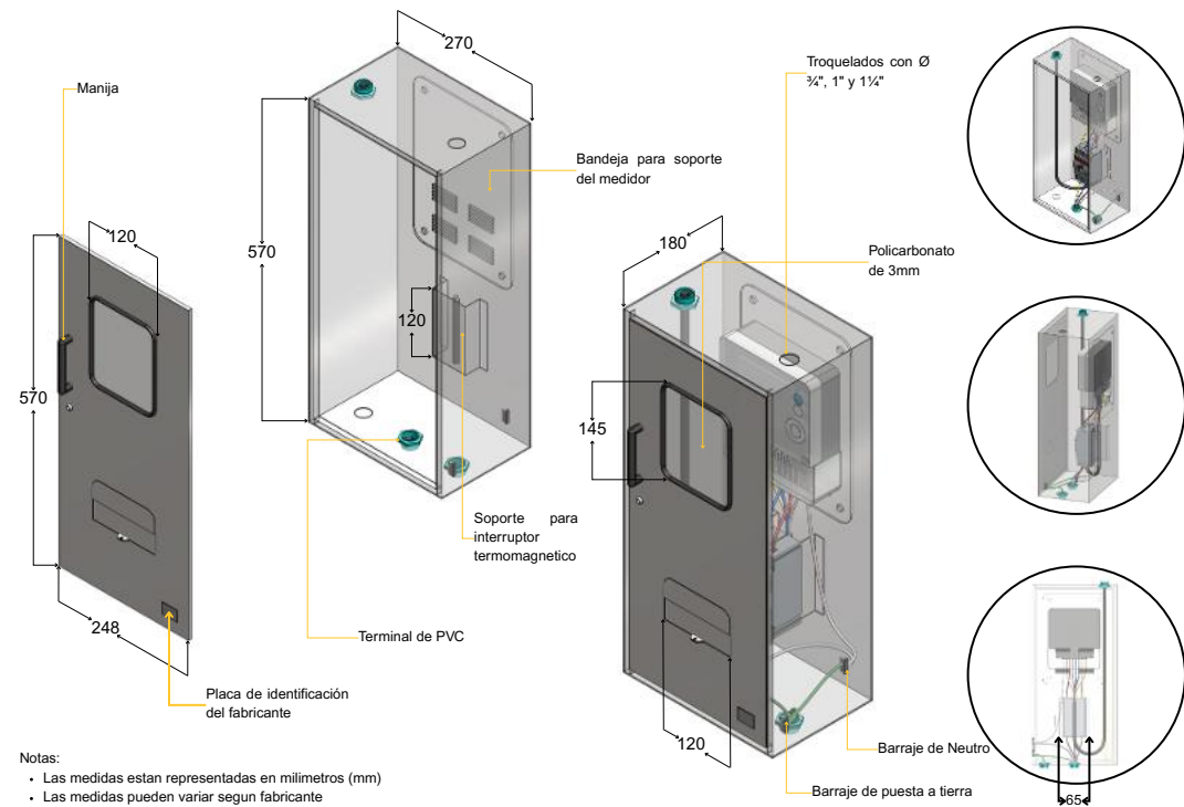
Figura 21. Detalle de gabinete de medida
