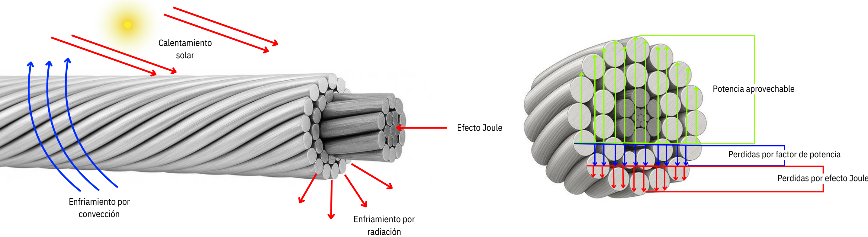
Figura 14. Fenómenos de calentamiento solar, efecto Joule y convección en conductores aéreos.
