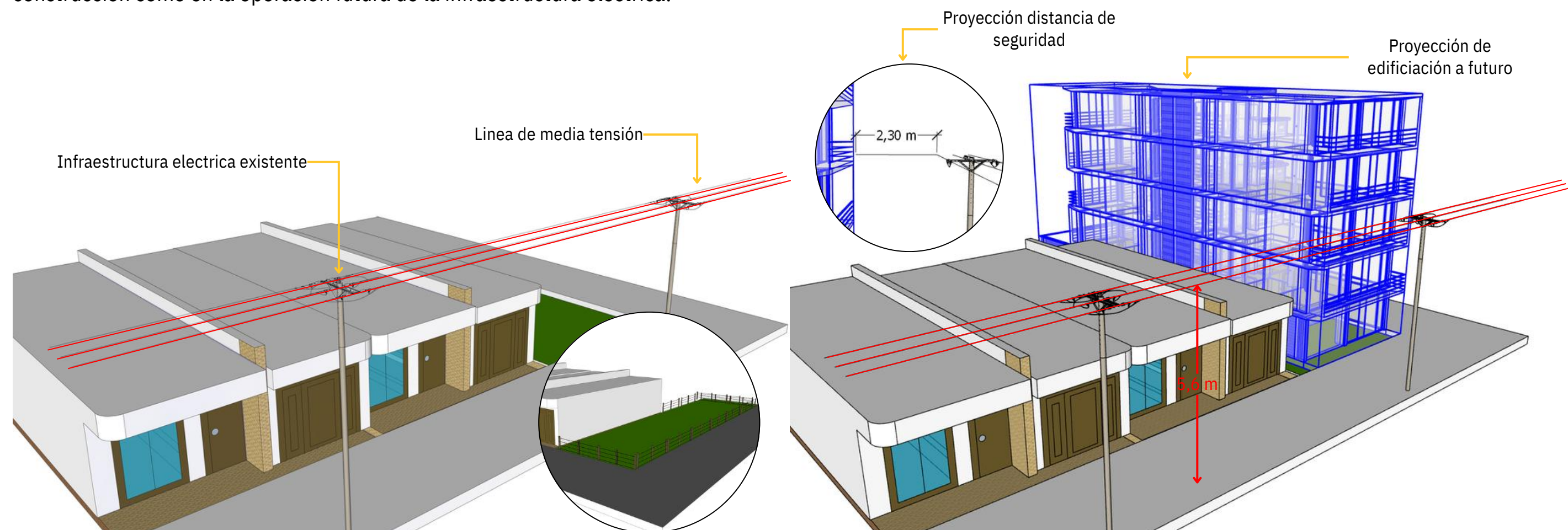
Figura 3. Distancias mínimas de seguridad en zonas con construcciones con infraestructura eléctrica existente.
