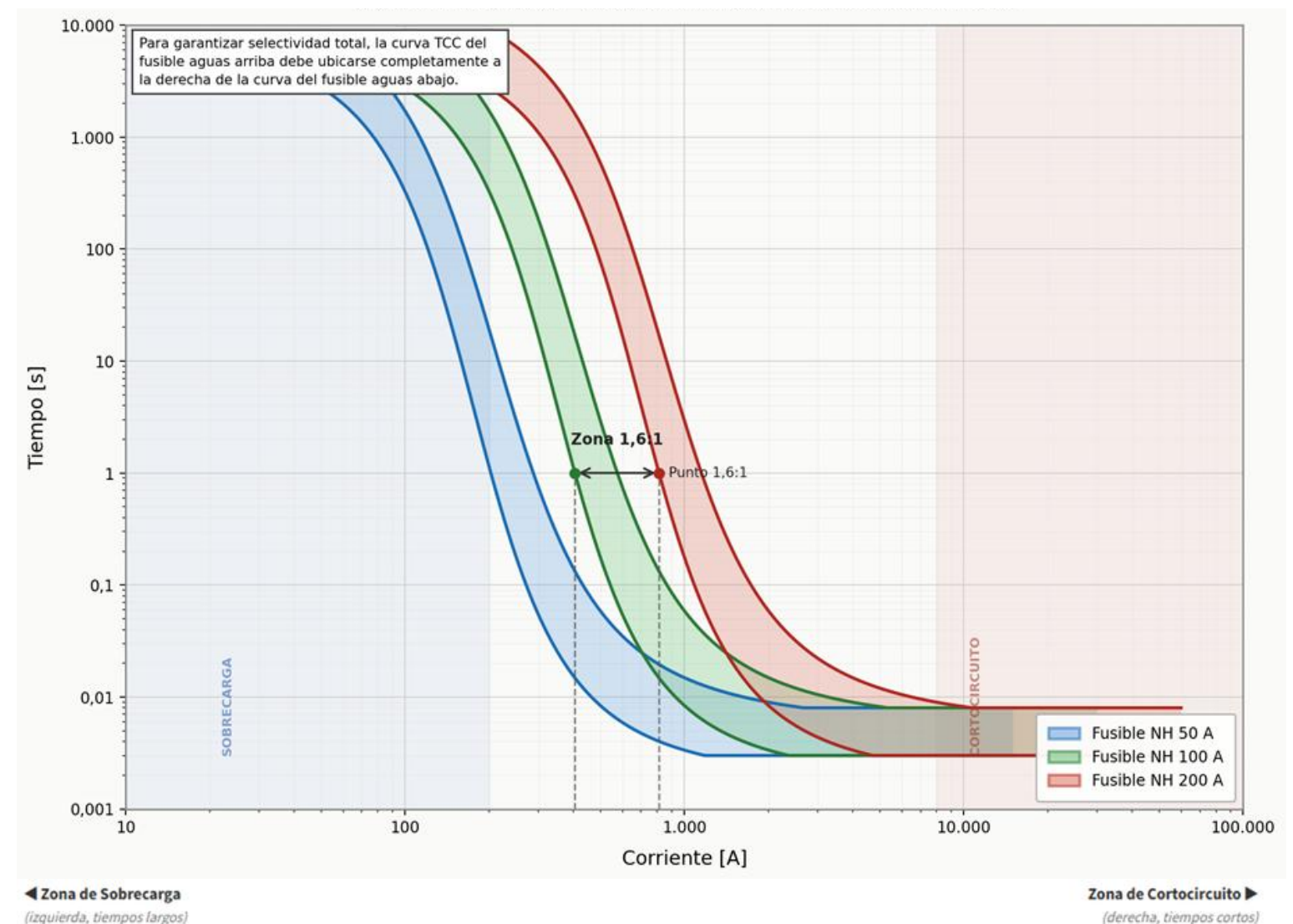
Figura 6. Curvas Características Tiempo-Corriente (TCC) de Fusibles NH
