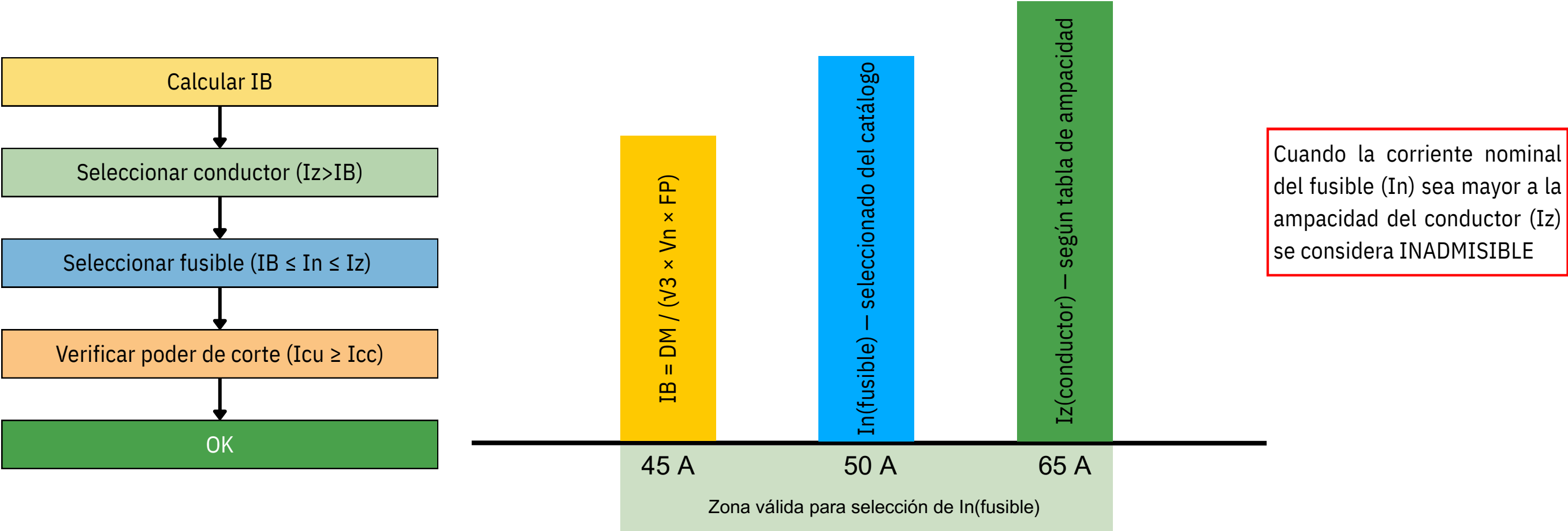
Figura 5. Esquema de Selección del Dispositivo de Protección
