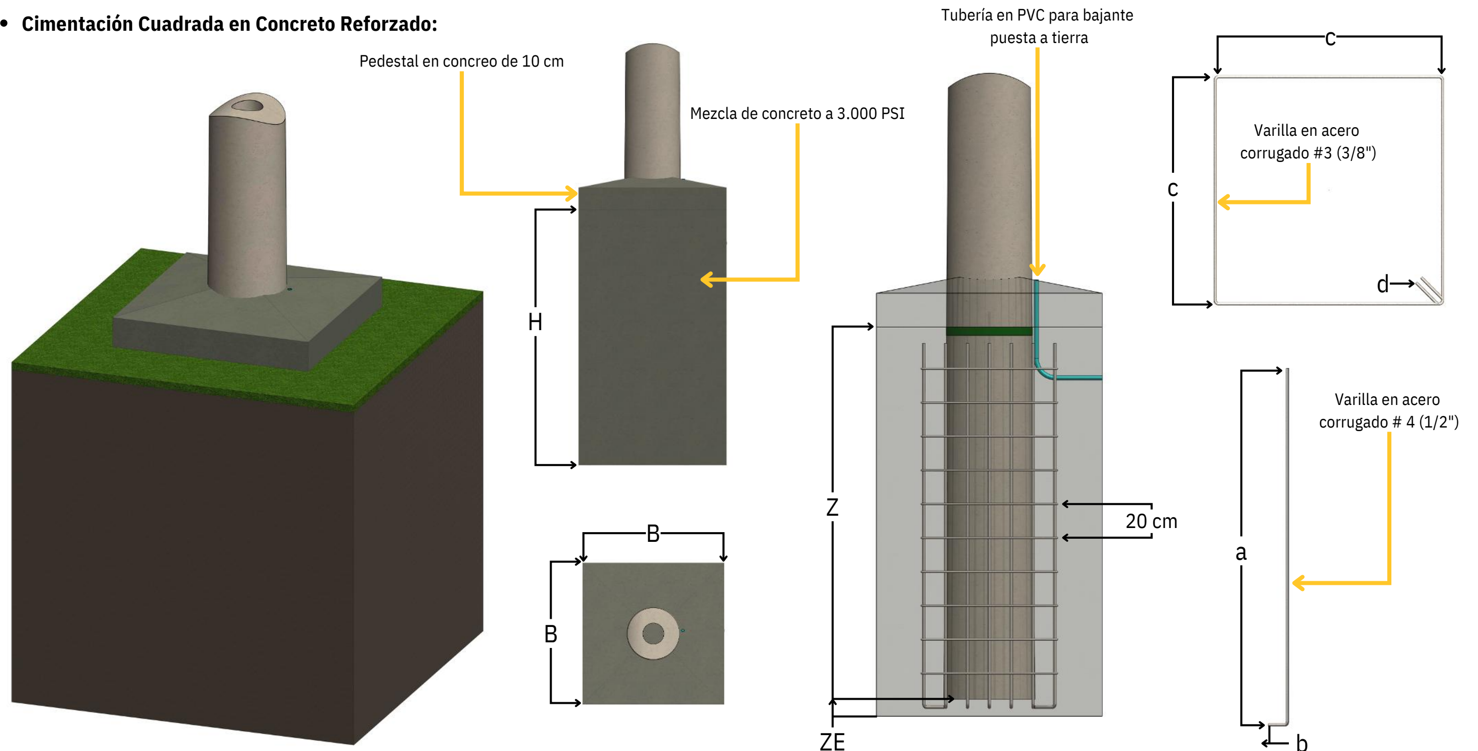
Figura 5. Geometría y Variables del Bloque de Cimentación Concreto Reforzada
