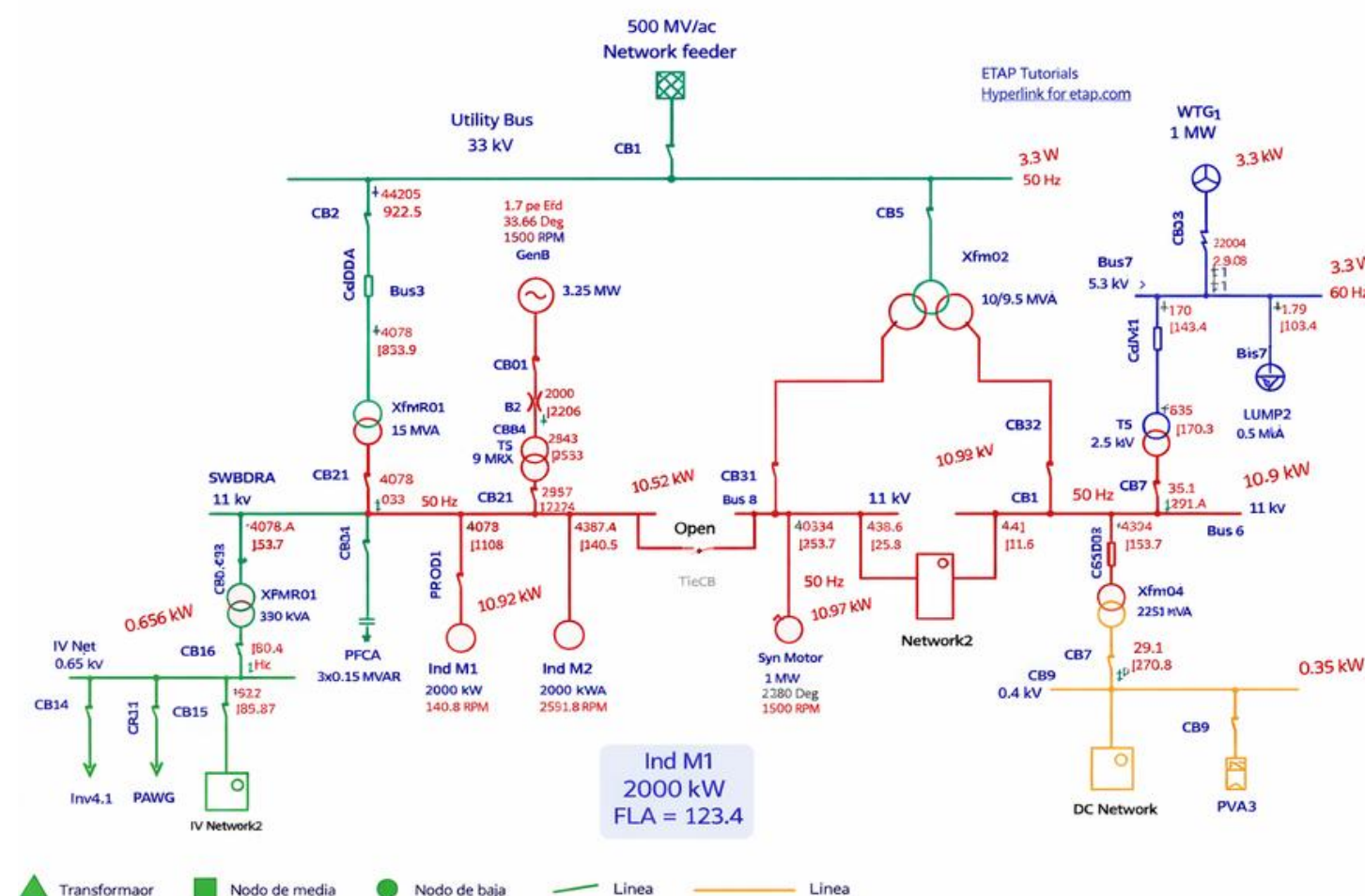
Figura 11. Ejemplo de simulación eléctrica utilizada en el estudio de conexión simplificado
