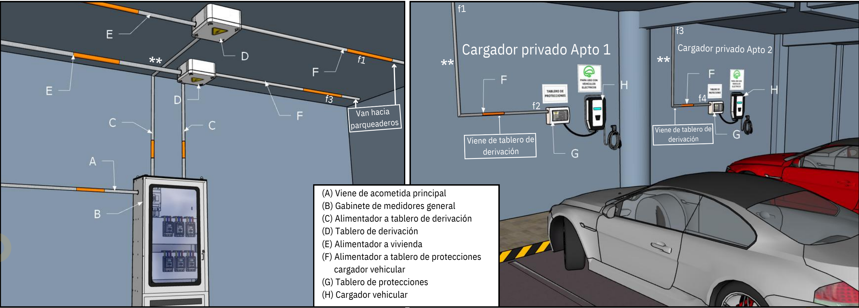
Figura 24. Representación conexión de estación de carga desde la caja de derivación de cada propietario.
