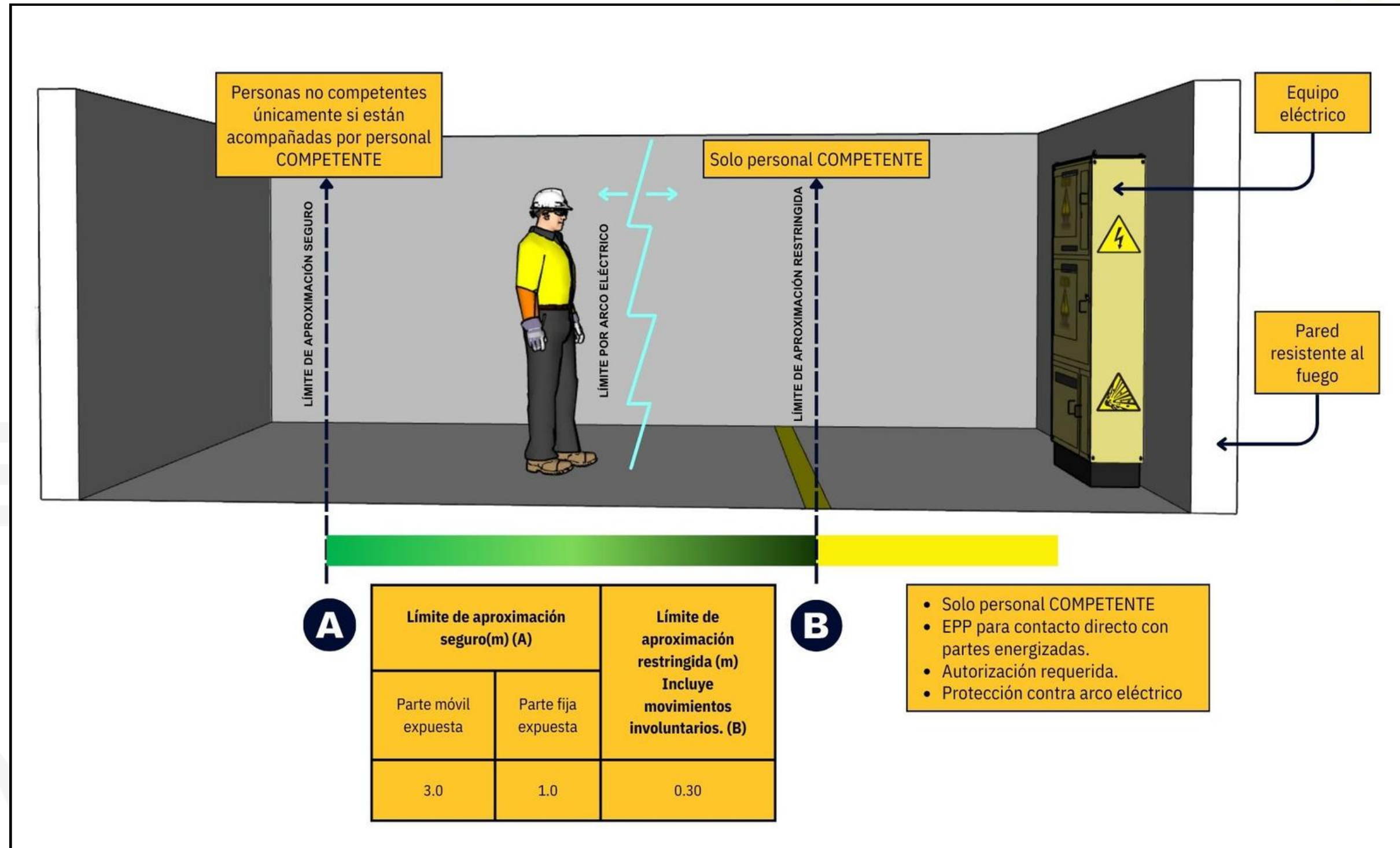
Figura 6. Distancias mínimas de aproximación
