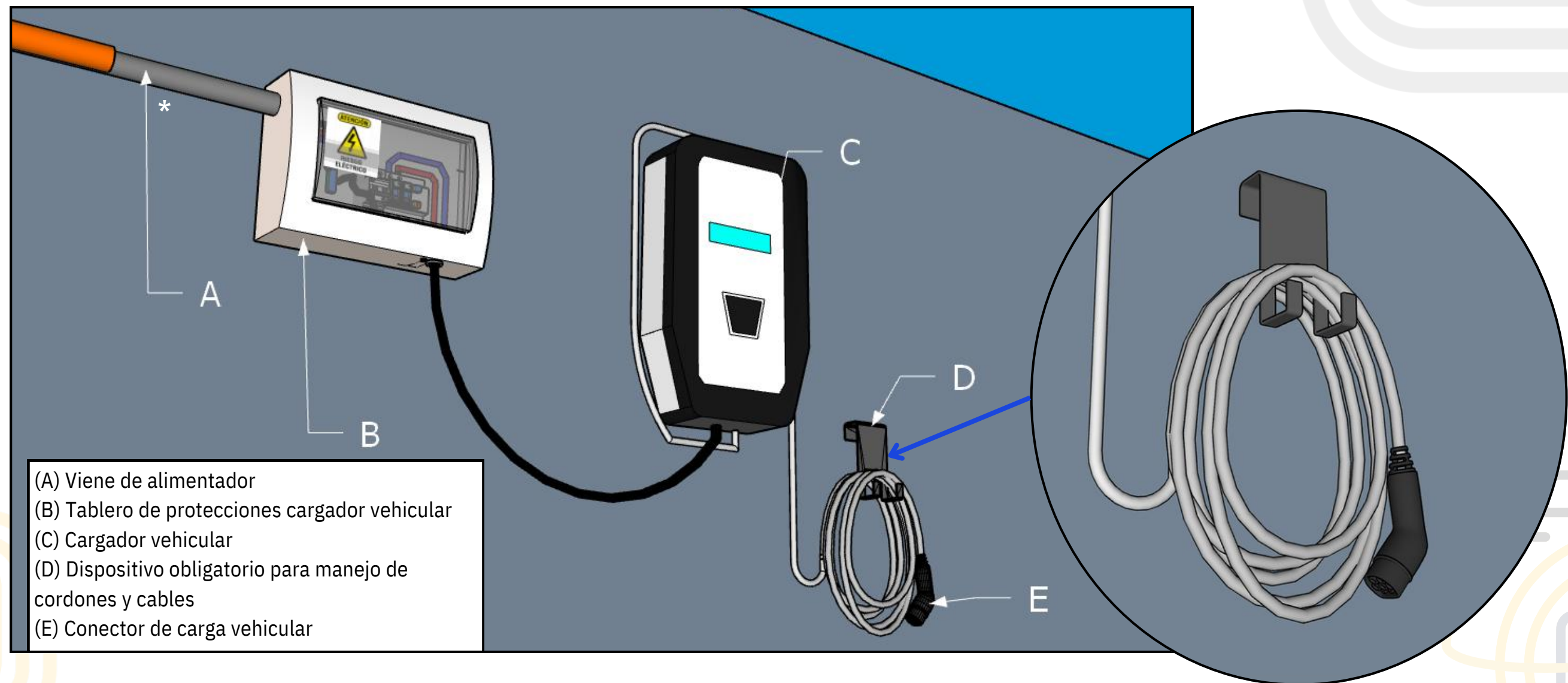
Figura 13. Demostración del dispositivo para el manejo de cordones y cables
