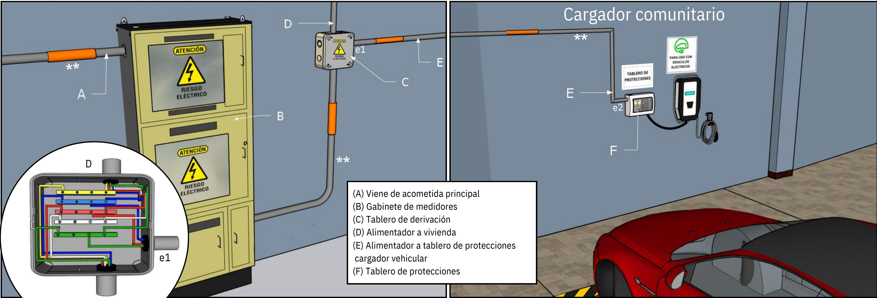
Figura 23. Representación conexión de estación de carga desde el medidor de áreas comunes.
