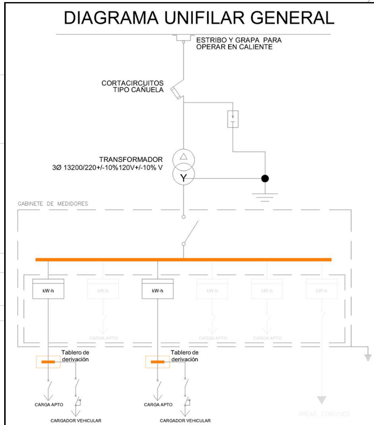
Unifilar 5. Unifilar de conexión de estación de carga desde la tablero de derivación de cada propietario.
