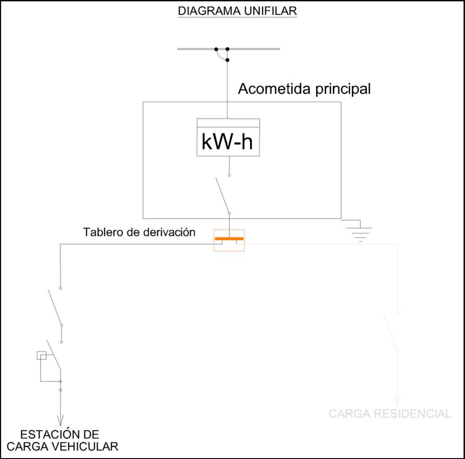
Unifilar 3. Unifilar de conexión de estación de carga (con tablero de derivación).
