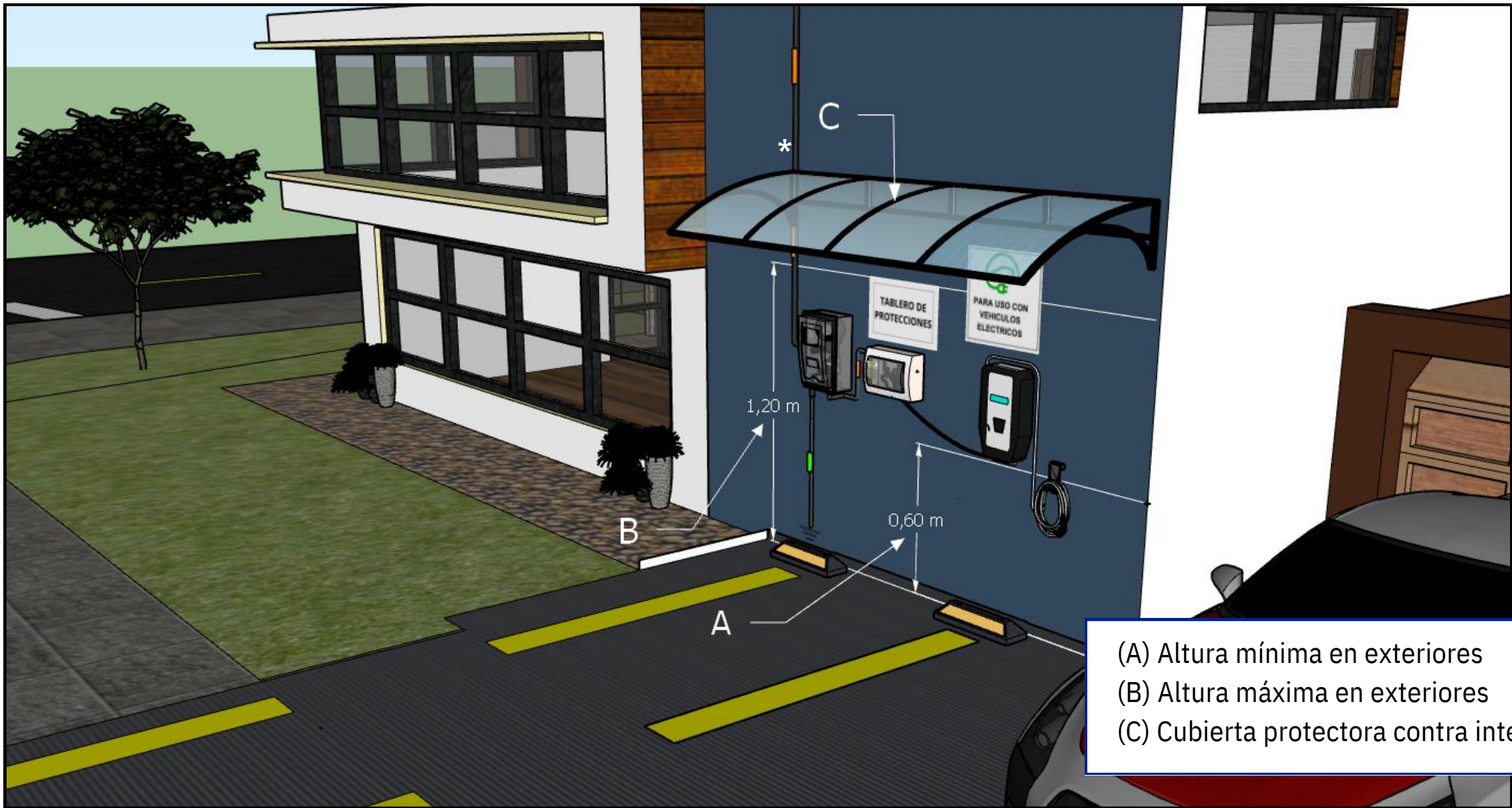
Figura 9. Ubicación de equipos de suministro y tablero de protecciones en exteriores
