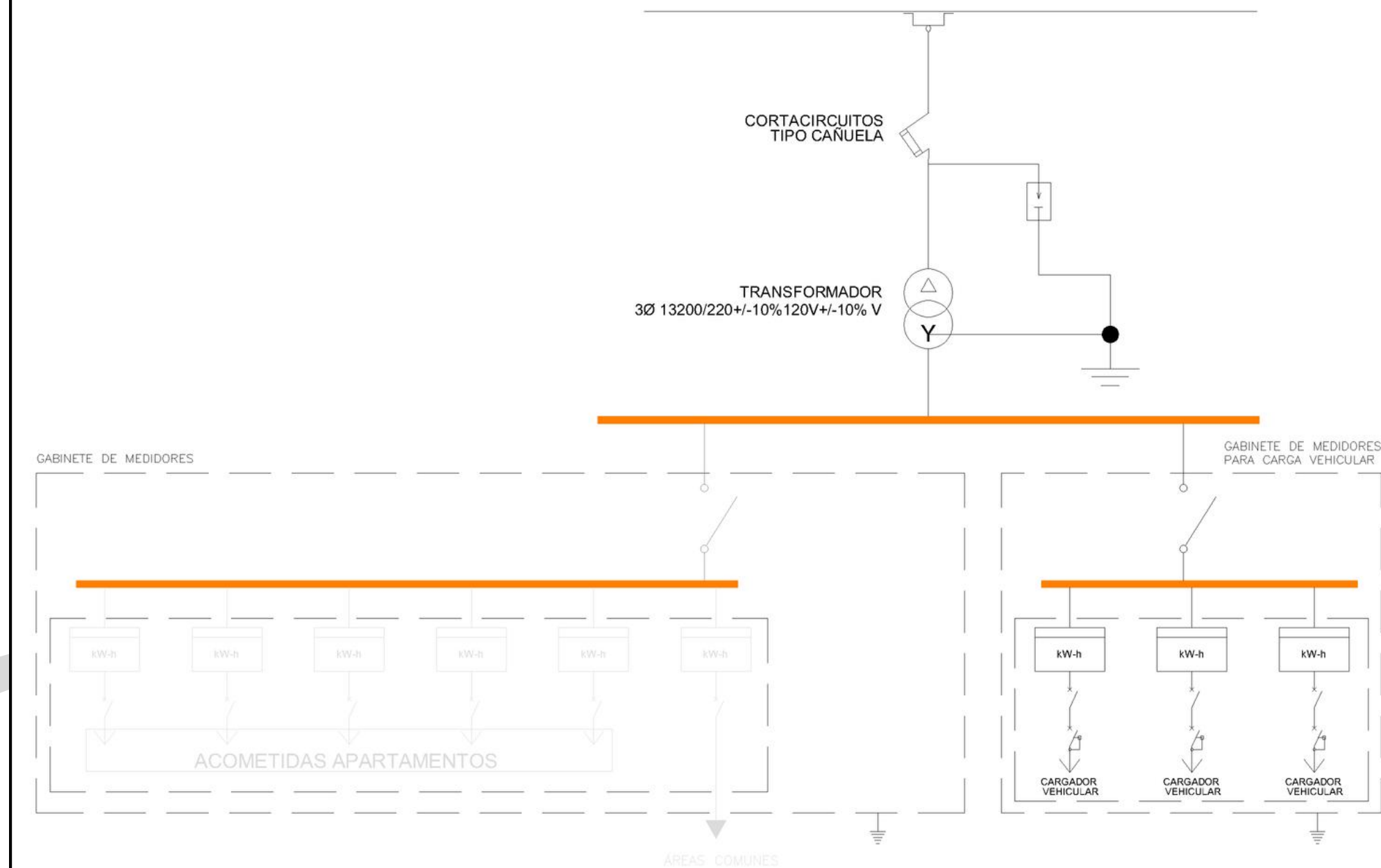
Unifilar 6. Unifilar de conexión de estación de carga con gabinete independiente
