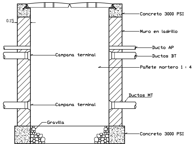
VISTA LONGITUDINAL
