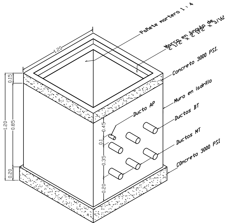
VISTA ISOMETRICA
