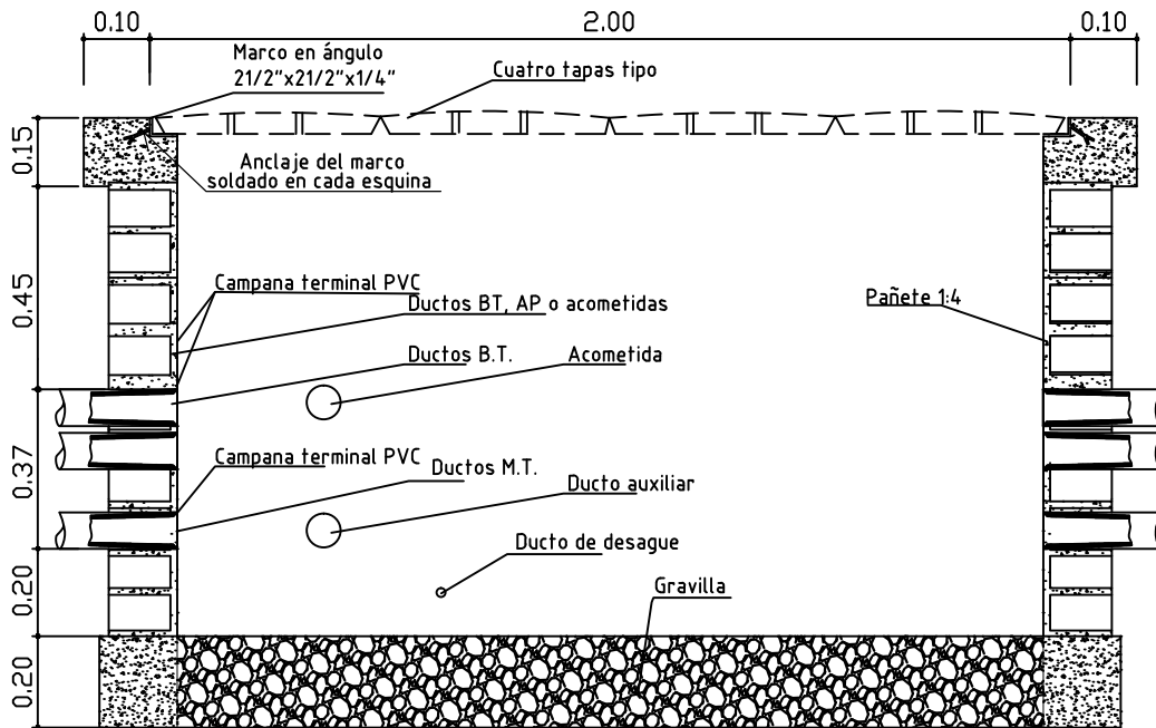
CORTE LONGITUDINAL
