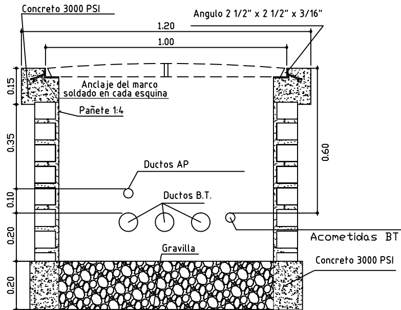
CORTE TRANSVERSAL
